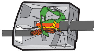
Зажим CAGE CLAMP®
